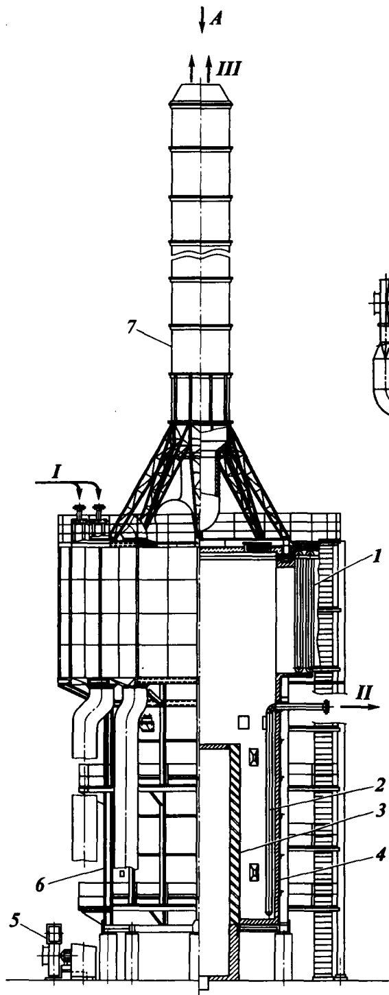
Рис. XXI-15. Конструкция печи типа КД4: 1 — змеевик конвекционных труб; 2 — змеевик радиантных труб; 3 — распределитель-распределитель; 4 — футеровка; 5 — воздуходувка; 6 — каркас; 7 — дымовая труба; 8 — воздухоподогреватель. Потoki: I — продукт на входе; II — продукт на выходе; III — дымовые газы
